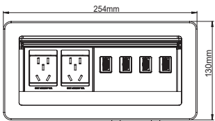
型号:CLB-B064-2100 配置:2个滑动电源 4个抽线结构
