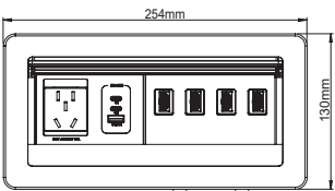
型号:CLB-B064-3100 配置:1个滑动电源 1个65W氮化镓适配器 4个抽线结构
