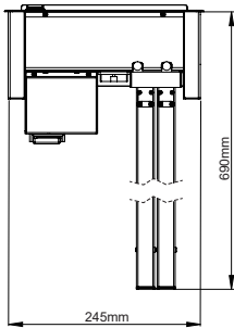
两根抽线、两D型模块
