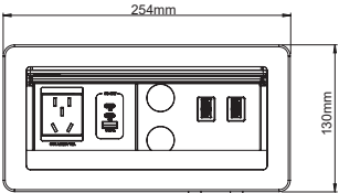
型号:CLB-B064-31D0 配置:1个滑动电源 1个65W氮化镓适配器 2个可选D型模块 2个抽线结构
