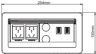
型号:CLB-B064-21D0 配置:2个滑动电源 2个可选D型模块 2个抽线结构
